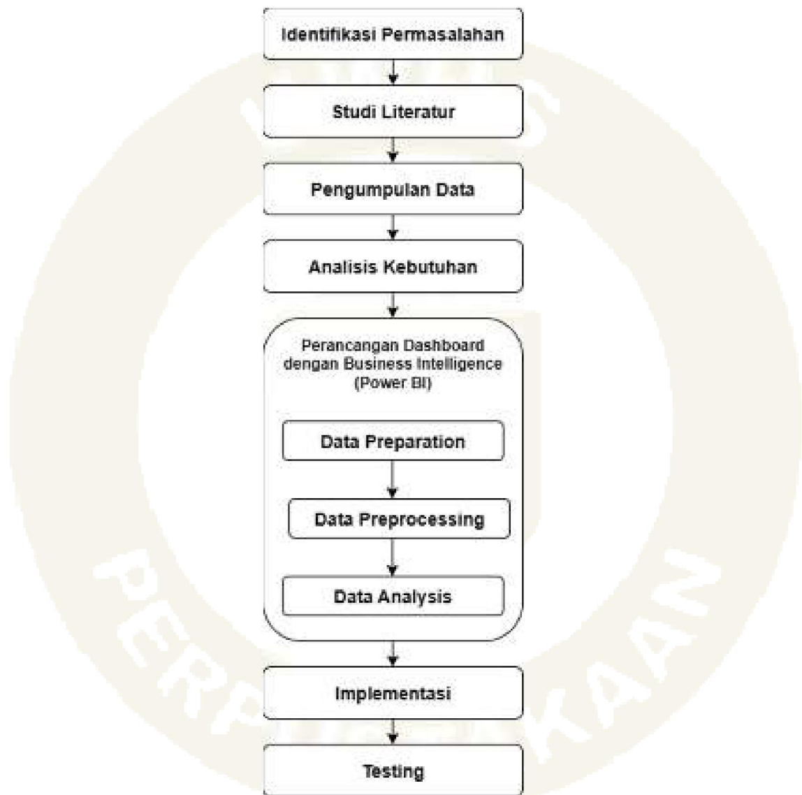
Gambar 3. 1 Kerangka Konsep
